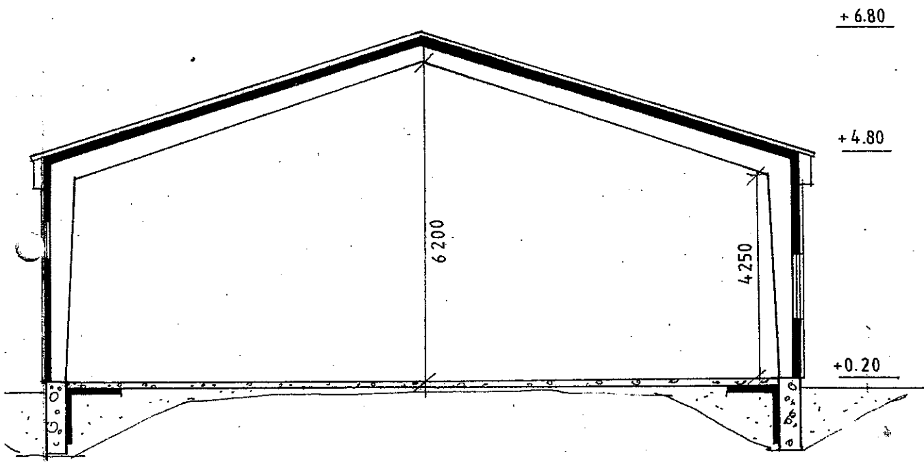
LEIKKAUS A-A
